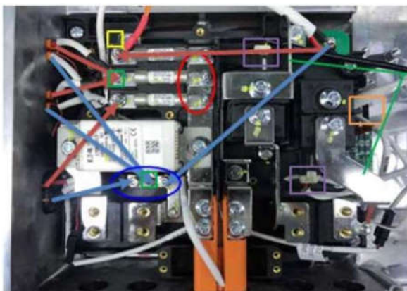
4.1.2 将高压线束、+16 线束、主铜压缩线束和电池加热线束的蓝色箭头安装在蓝色框内。在红色框内。 将高压线束、+16 线束、主铜压缩线束和电池加热线束的蓝色箭头安装在蓝色框内。示意如图 4.7.6-2
