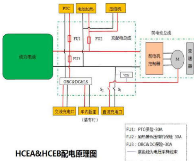
图 3-2 HCE 高压系统原理框图
